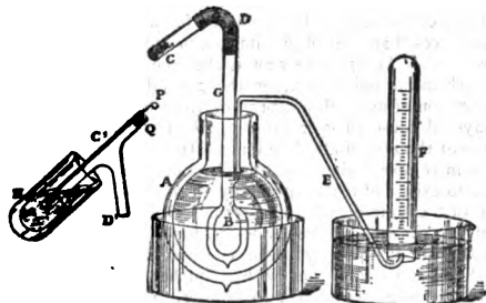
FIG. 13.—Calorimetric Apparatus.
