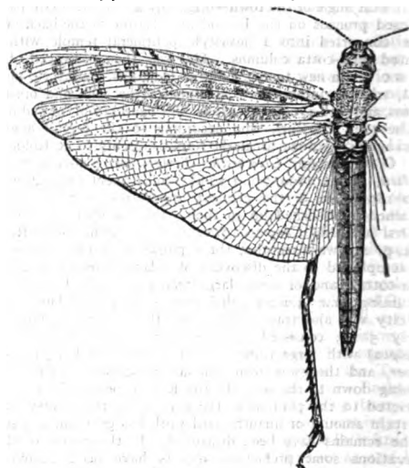
FIG. 2.— Acridium peregrinum .
