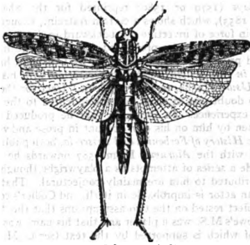
FIG. 3.— Caloptenus italicus .
