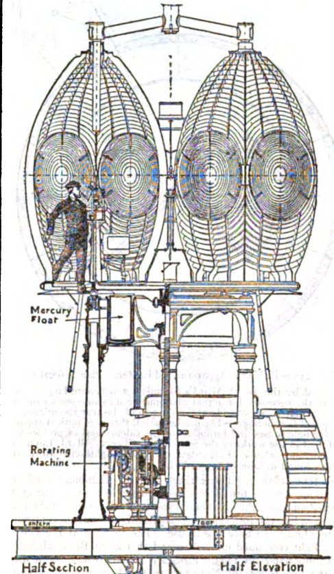
FIG. 43.—Le Vierge Apparatus.
